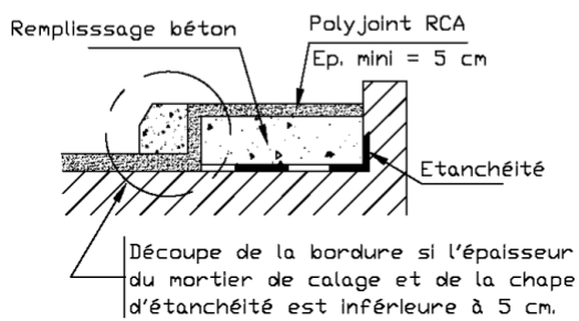
Coupe schématique C-D
