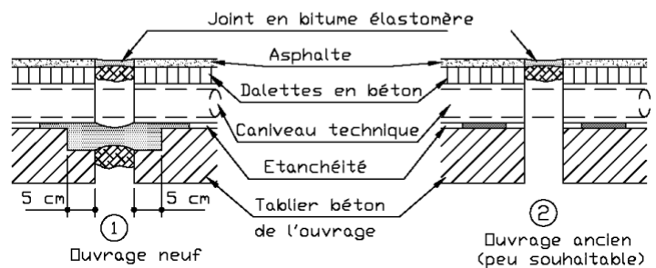
Coupe de la feuillure A-B
