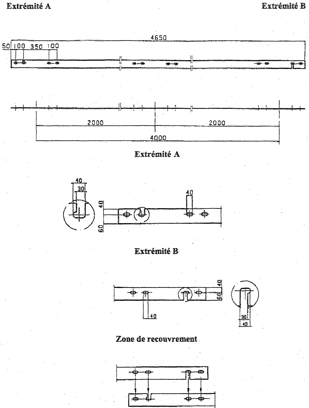
Figure 4: renfort métallique 4650 x 100 x 5
