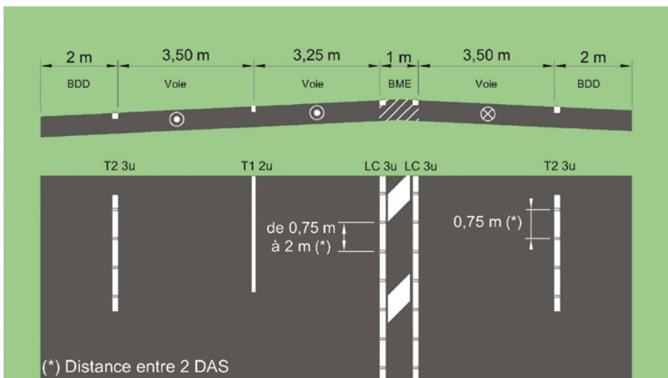
Figure 22 : Profil en travers et vue en plan d'une route à 3 voies affectées, avec BME équipée de hachures et d'alerte sonore
