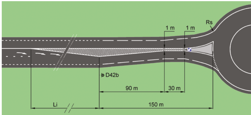
Figure 47 : Approche d'un giratoire depuis une artère interurbaine, avec entrée à 2 voies 170
