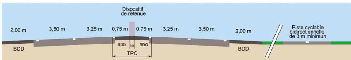
Figure 13 : Profil en travers d'une artère interurbaine limitée à 90 km/h
