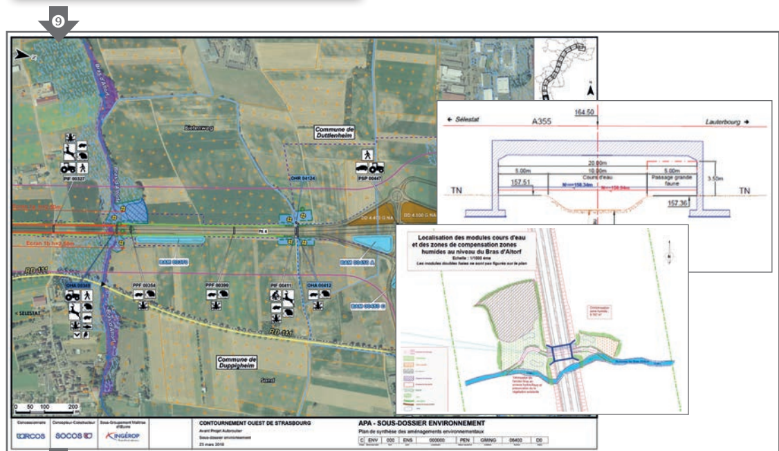
Exemple des pièces transmises dans le cadre d'une étude d'avant-projet autoroutier. Plan masse des mesures prévues au droit du franchissement du Bras d'Altorf. Profil en travers type de l'ouvrage du cours d'eau et représentation schématique des aménagements écologiques proposés au droit du cours d'eau. Étude d'avant-projet autoroutier du contournement Ouest de Strasbourg. SOCOS/SINBIO. 2018.
