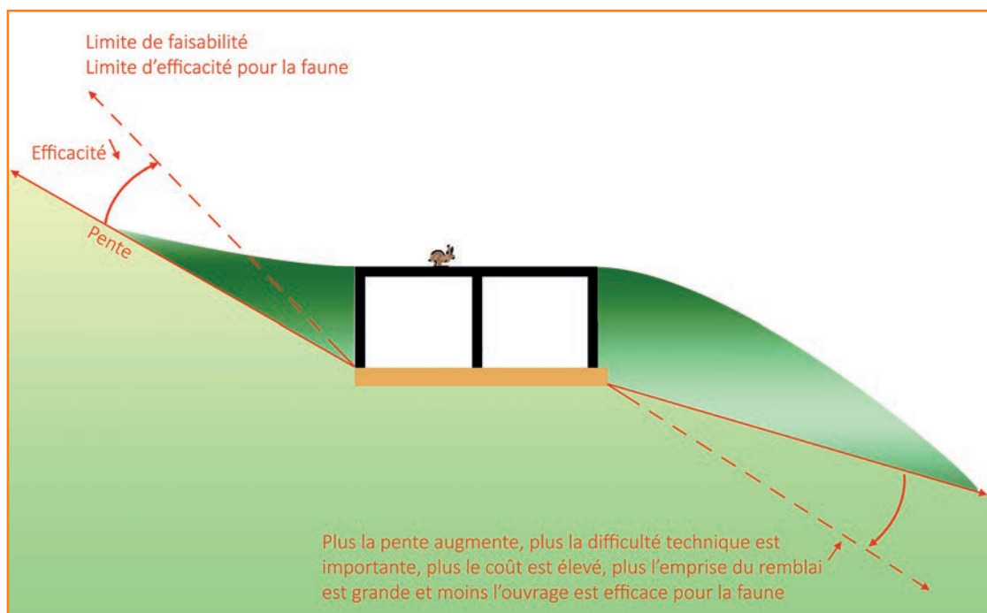
6 Représentation schématique d'une infrastructure dont le profil est mixte et où la difficulté d'aménagement est généralement liée à l'importance de la pente des talus situés de part et d'autre de l'infrastructure. Source : Cerema.
