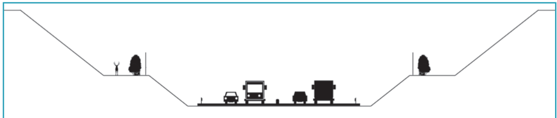
③ Schéma d'aménagement de risbermes* dans les déblais importants permettant de constituer une zone favorable aux déplacements de la faune et d'implanter les clôtures. Source : Cerema.
