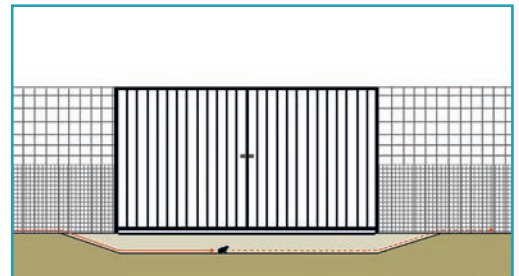
7 Schéma d'implantation d'un caniveau au droit d'un portail. Source : Cerema.
