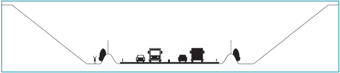
② Schéma d'aménagement de merlons de protection en zone de déblais assurant la tranquillité des dépendances pour la faune terrestre. Source : Cerema.
