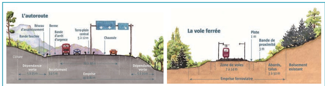
Profil en travers d'une autoroute et d'une voie ferrée.
