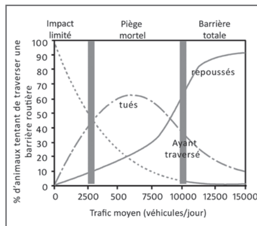
Effet de fragmentation des infrastructures routières en fonction du trafic moyen journalier. Source : Rapport COST 341 adapté de Seiler, 2003.
