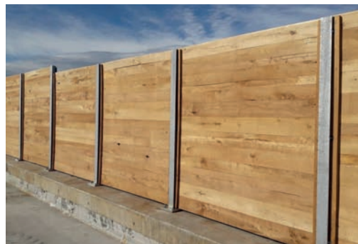
16 Écran du passage à faune de La Buisse (A48 – Réseau APRR), réalisé en robinier faux-acacia non traité chimiquement. Le bois a été prélevé localement sur des dépendances autoroutières et transformé à proximité (sciage et fabrication des panneaux). Afin de déterminer la classe de résistance de ce bois pour dimensionner les panneaux, une sélection de planches a fait l'objet de tests de flexion. Source : APRR.
