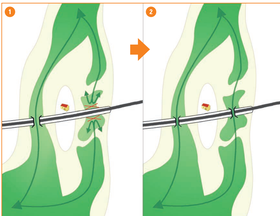
10 Schéma représentant deux continuités écologiques proches et reliées pouvant justifier la création d'un ouvrage de franchissement de taille réduite sur chacune d'entre elles (2) plutôt qu'un seul ouvrage de plus grande taille (1). Source : Cerema.
