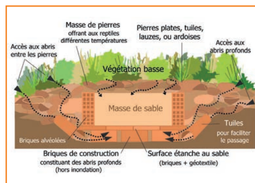
30 Exemple d'un abri multifonctionnel pour reptiles. Source : dessin de C. Houel, d'après D. Guerieau.
