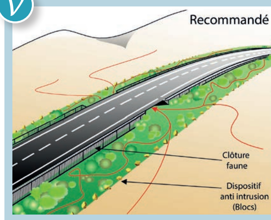
1 Schéma d'implantation des clôtures permettant à la faune d'accéder aux dépendances vertes et d'être guidée jusqu'aux ouvrages de franchissement. Source : Cerema.
