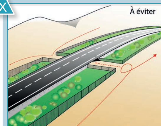
3 Schéma d'implantation des clôtures ne laissant pas les dépendances vertes accessibles à la faune et dont la disposition à l'approche de l'entrée de l'ouvrage crée un effet couloir défavorable au passage de la faune. Source : Cerema.
