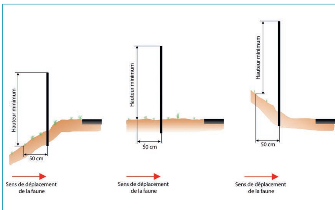
Détermination de la hauteur minimale de la clôture selon la configuration du terrain.
