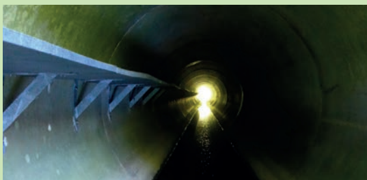
Banquette en plastique recyclé de 50 cm de largeur sur 65 m de long et un tirant d'air de 70 cm. Coût : 15 000 € TTC (2013). RN137 (DIRO). Source : Cerema.
