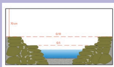
Schéma de principe d'une banquette en gradins. Source : Cerema.
