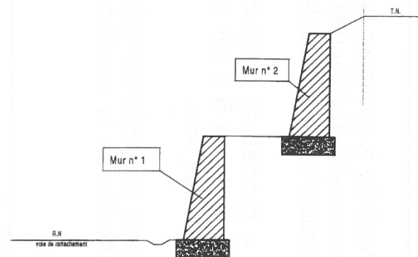
Schéma de principe de soutènement en terrasse des terrains surplombant la voie
