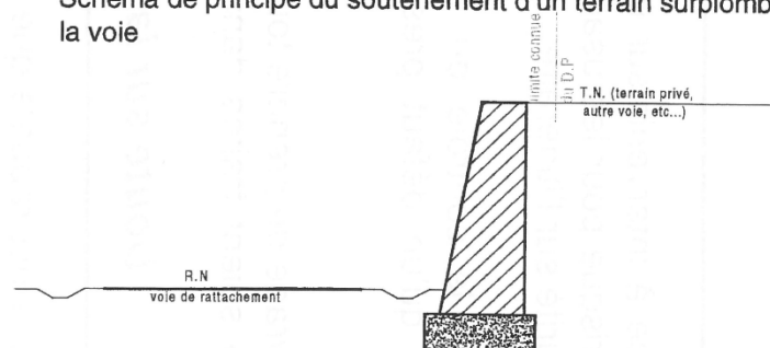
Schéma de principe de soutènement en terrasse des terrains surplombant la voie
