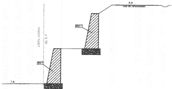
Schéma de principe d'un soutènement en terrasse de la voie
