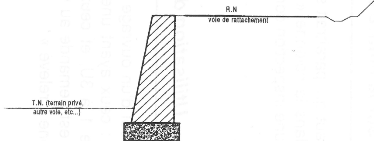
Schéma de principe d'un soutènement direct de la voie
