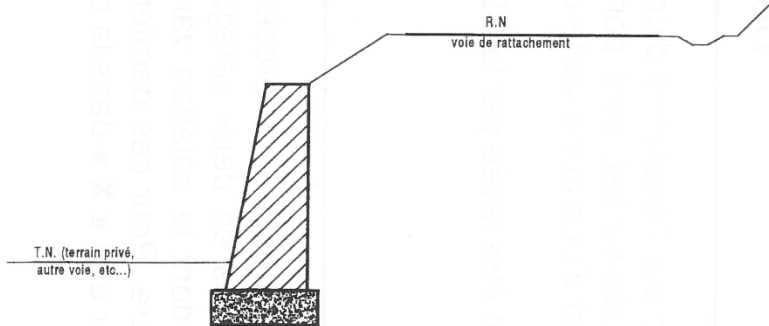
Schéma de principe d'un soutènement en pied de talus de la voie
