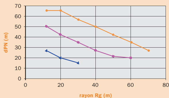
Graphique 2 : limite d'utilisation d'un feu en entrée
