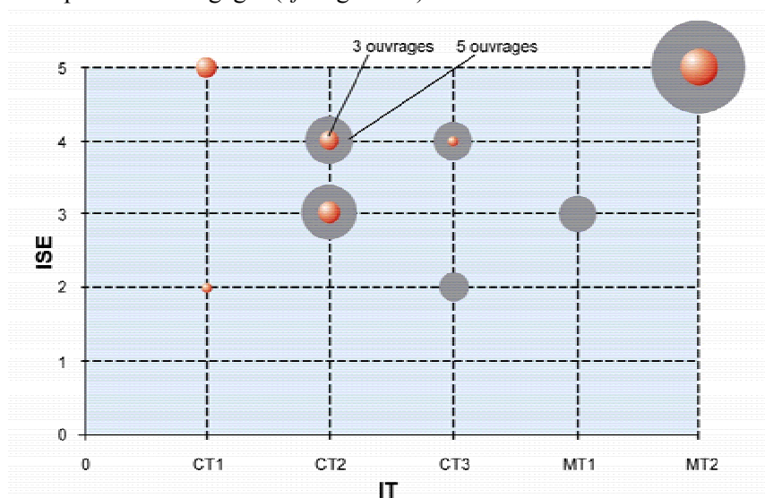
Figure 13 – Exemple de représentation sur un graphe croisé des ouvrages devant être réparés (en gris) et identification de ceux proposés dans le programme de réparation (en rouge).
