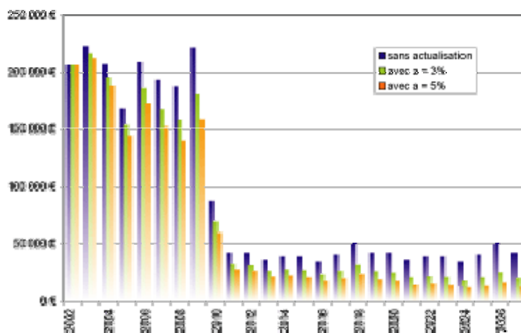
Figure 24 – Cas 1, comparaison des coûts annuels de maintenance avec ou sans prise en compte d'une actualisation des coûts (voir tableau 15).
