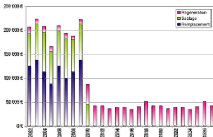
Figure 21 – Cas 1, patrimoine peu entretenu (voir tableau 12).
