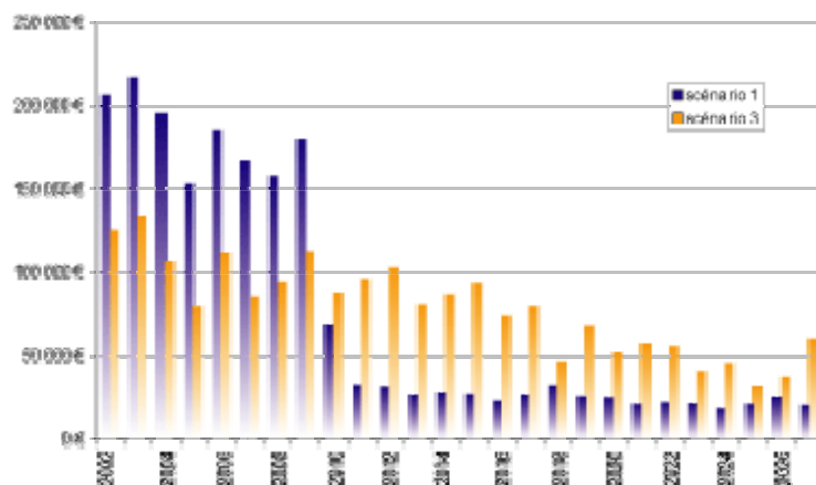
Figure 25 – Cas 1, comparaison entre deux politiques d'intervention avec un taux d'actualisation de 3 % appliqué aux deux scénarios. (voir Tableau 16).
