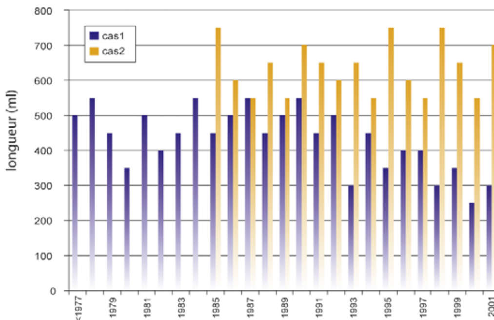
Figure 20 – Répartition du linéaire de dispositifs de retenue en fonction de la date de la dernière intervention de maintenance pour les cas 1 et 2.
